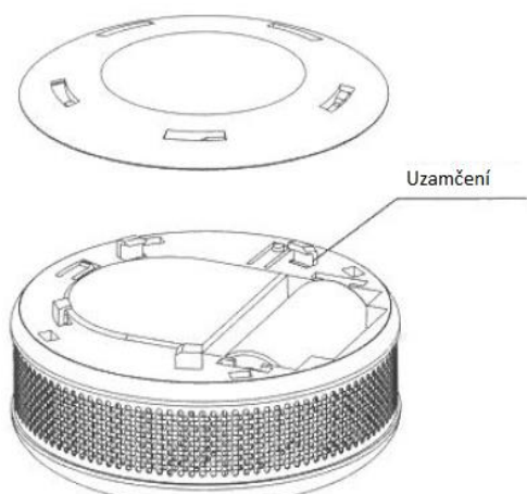
Obr. 3 – Pohled zespodu s instalovanou baterií
