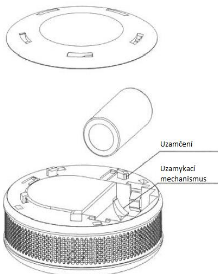
Obr. 2 – Pohled zespodu bez instalované baterie
