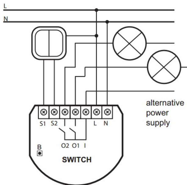
Obr. 1 Zapojovací schÄ½mata modulu dvojitého spínaÄ½e
